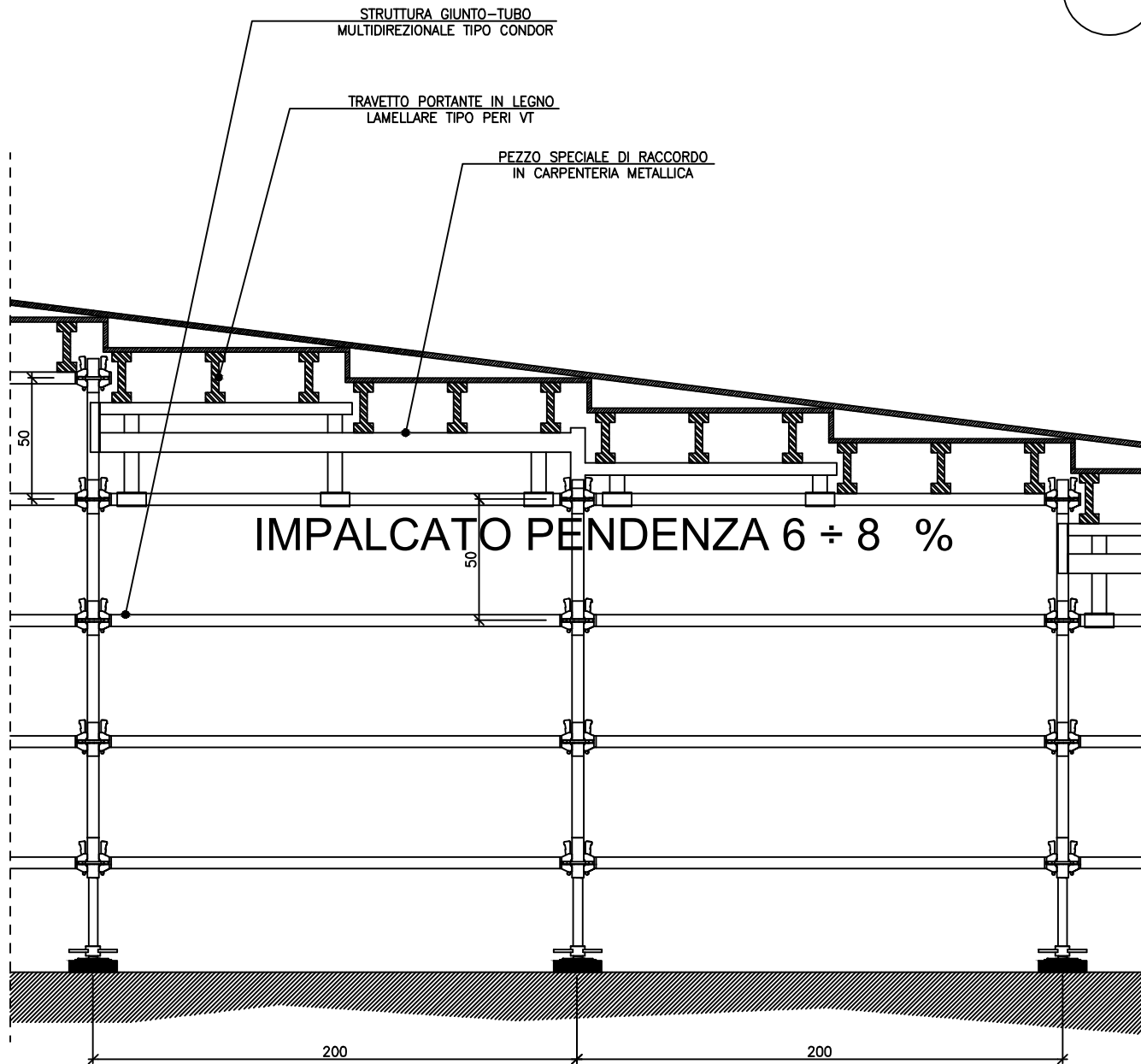
DETTAGLIO C 01.A - SEZIONE TIPICA STRUTTURA DELLA GRADONATA RAPP. 1:20
