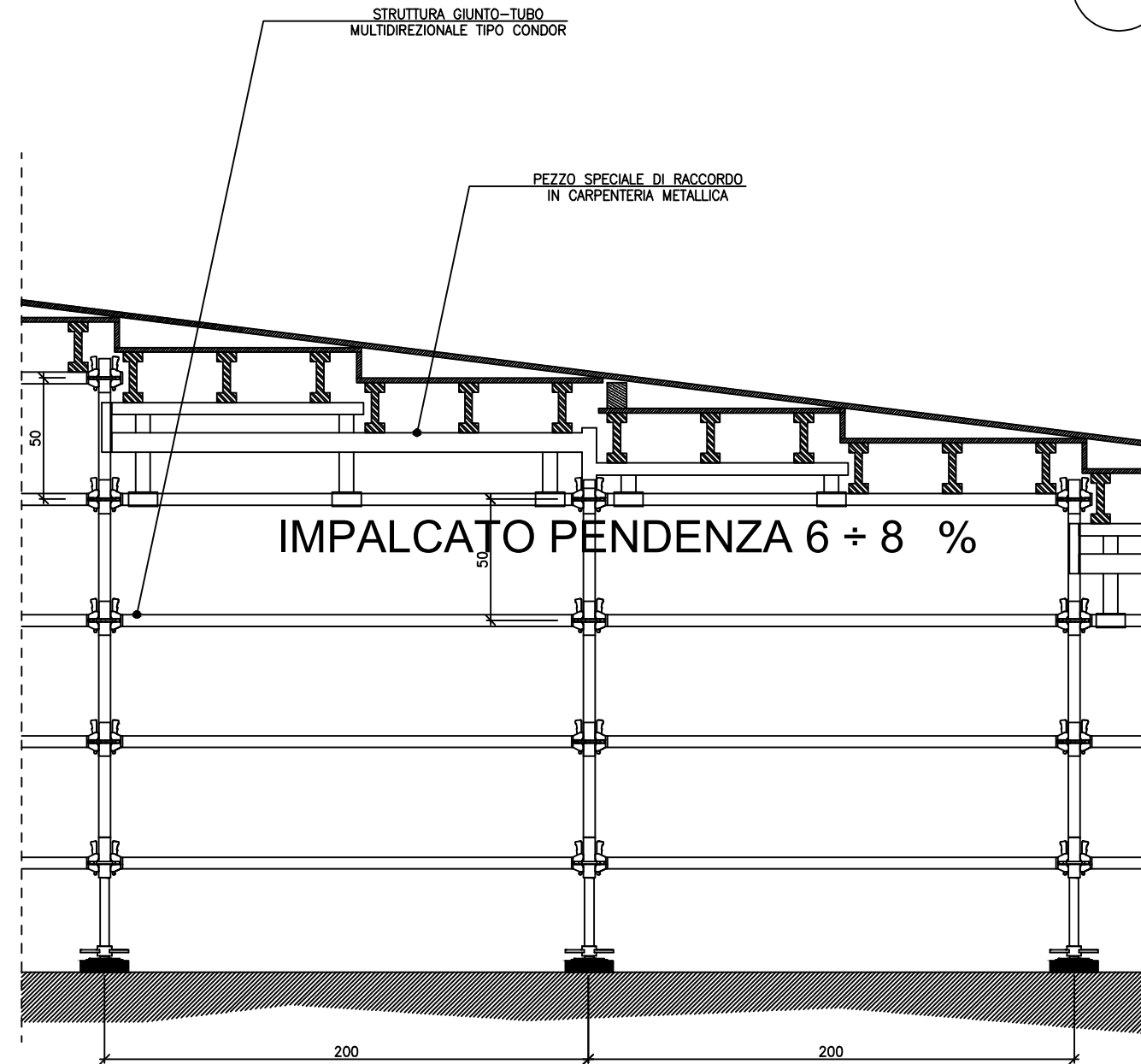
DETTAGLIO C 01.B - SEZIONE STRUTTURA DELLA GRADONATA - DOPPIA ALZATA RAPP. 1:20
